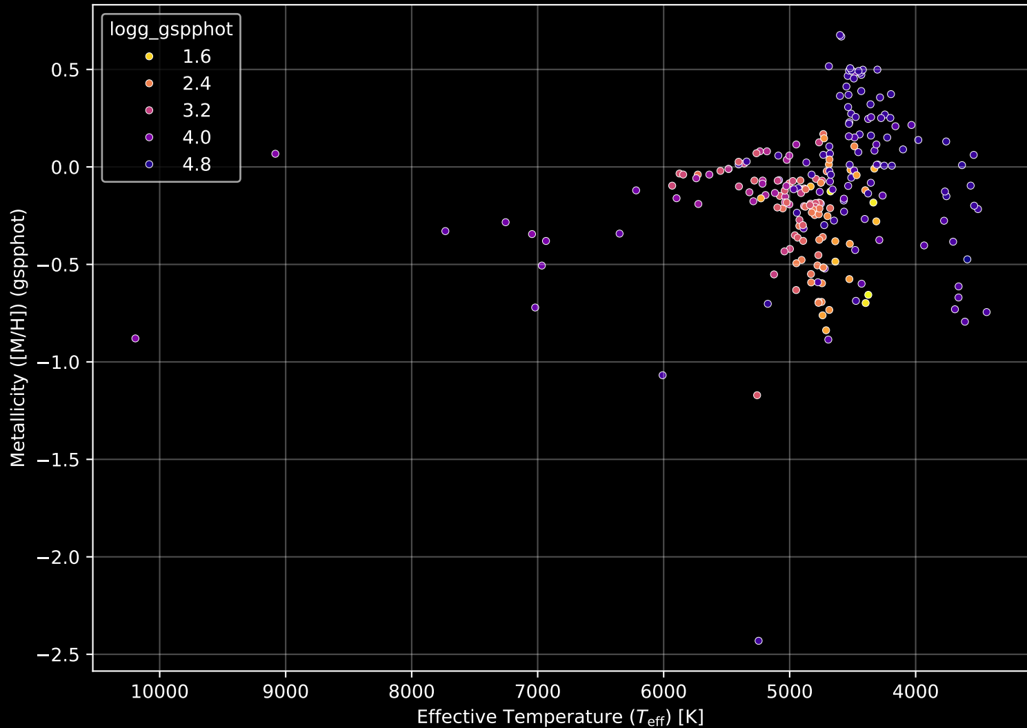
APOGEE DR17 Field: [148+31_btx] Stellar Population Parameters (n= 231)
